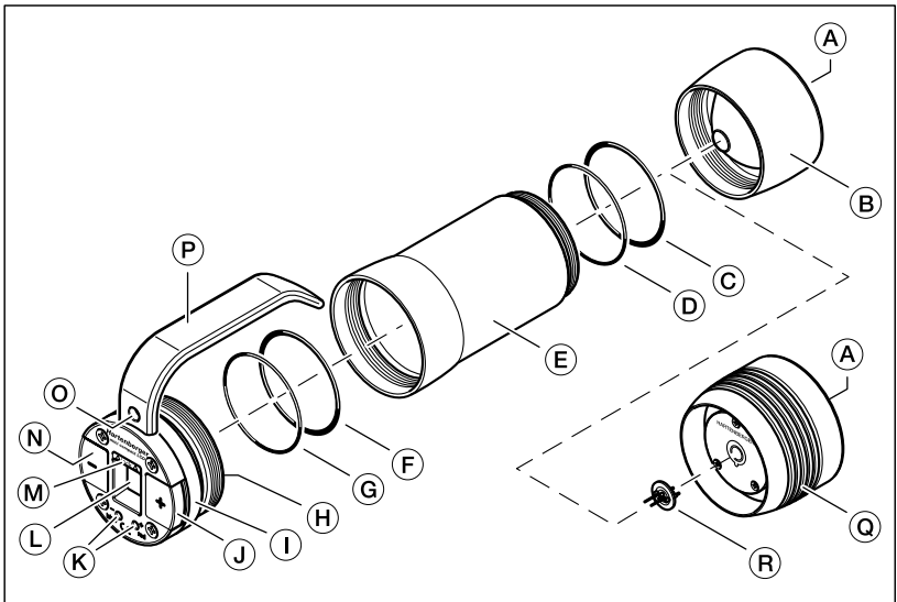
Abb. 1: Gehäuse
