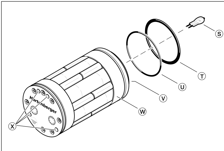
Abb. 2: Akkueinheit
